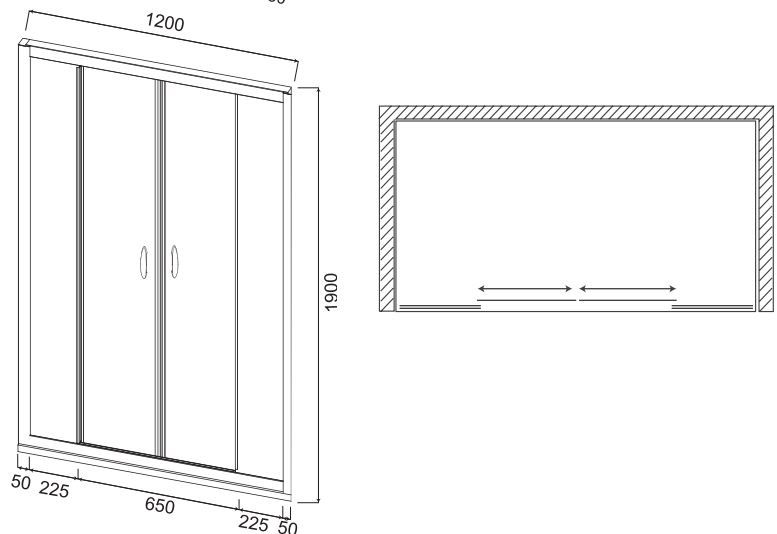
Душевая дверь в нишу Bliss Solo Twin
