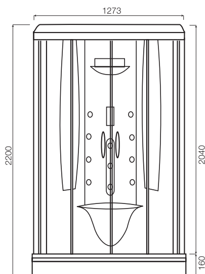
Гидромассажная кабина Bourgeois с паром
