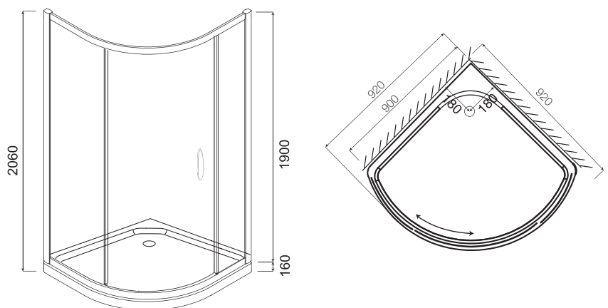
Душевой уголок Bliss Slide 3/4
