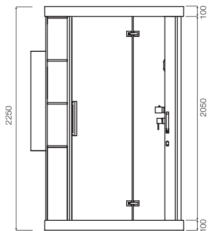
Гидромассажная кабина Awe, свободностоящая
