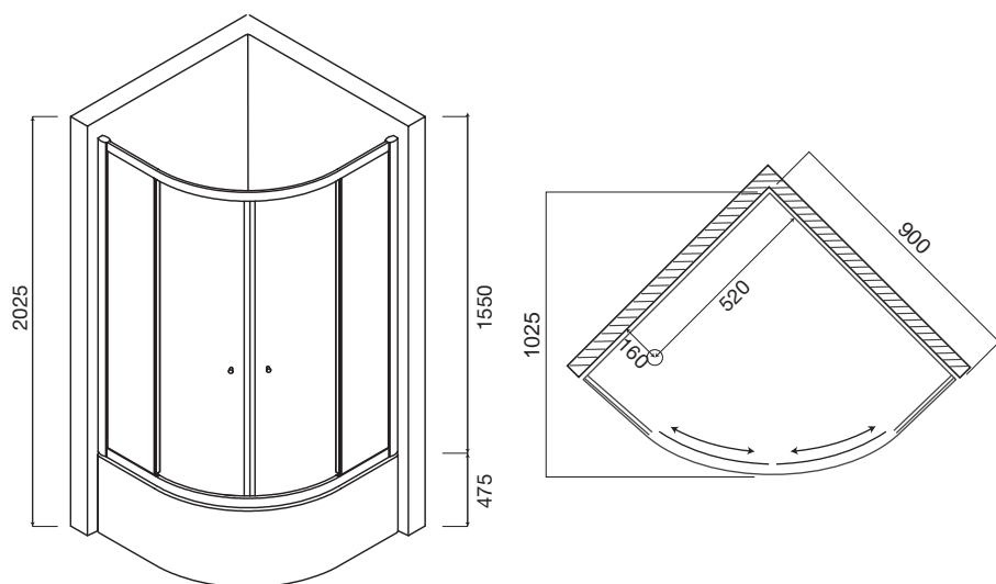
Душевой уголок Sense Deep, 90x90
