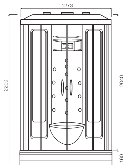
Гидромассажная кабина Sense 6 с паром
