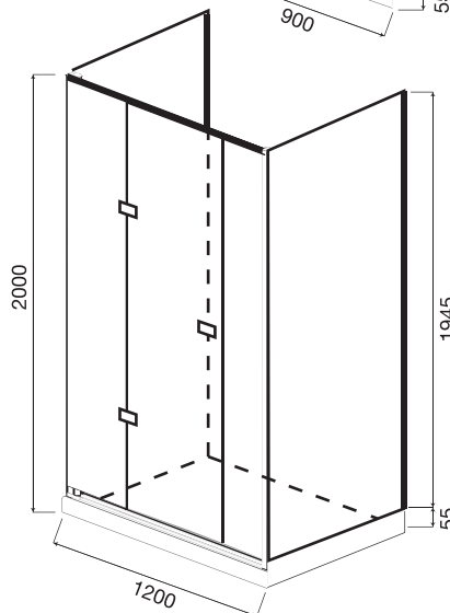
Душевой уголок Tender Square Wall 120
