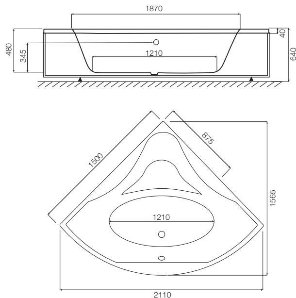
Акриловая ванна с гидромассажем, Bliss 150x150
