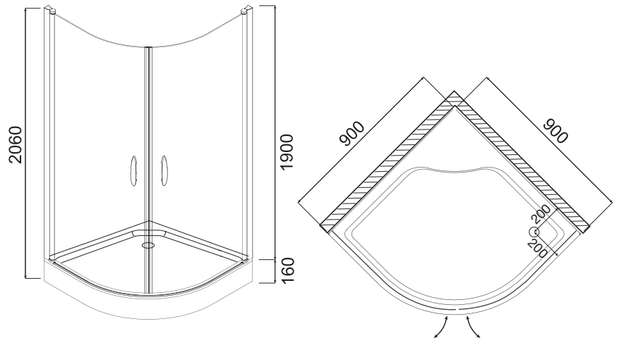
Душевой уголок Bliss full Swing, 90x90
