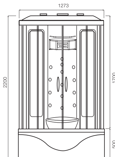
Гидромассажная кабина Sense Deep 6 с паром
