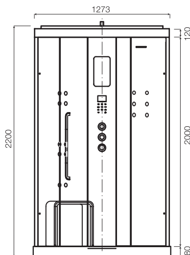
Гидромассажная кабина Inspire 90 с AMPM system и паром
