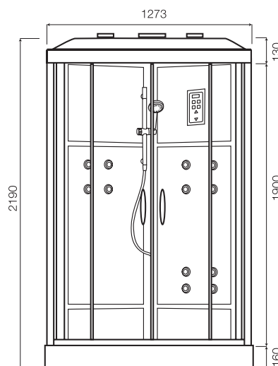
Гидромассажная кабина Joy
