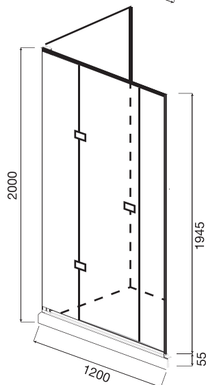
Душевой уголок Tender Square Corner 120
