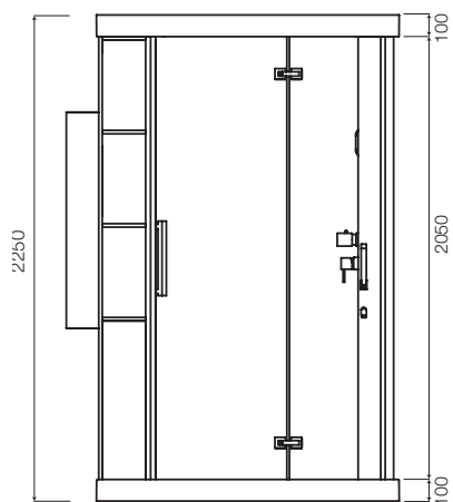
Гидромассажная кабина Awe, пристенно- фронтальная
