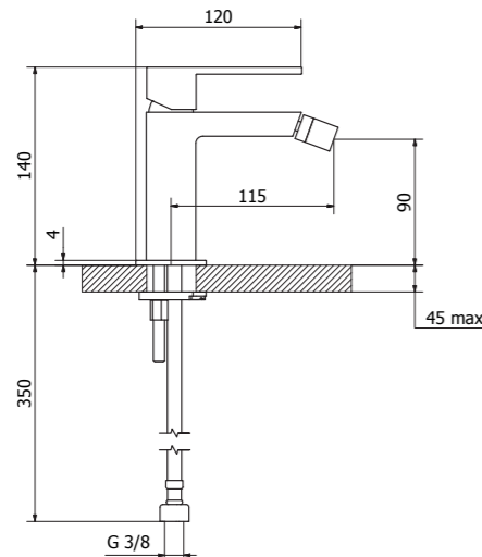
8G401 Bidet mixer
