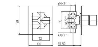
KVANT 4 vie deviatore Built-in 4-way diverter Девiator 4х позиционный
