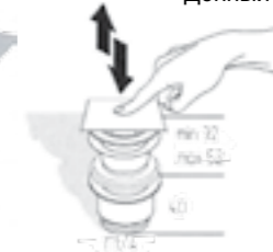
Scarico senza troppopieno Pop-up waste without overflow Донный клапан без перелива
