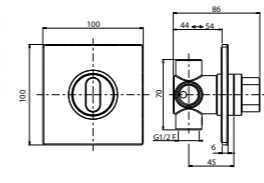
FORTIS 3 vie deviatore Built-in 3-way diverter Девiator 3х позиционный
