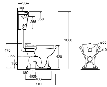
Vaso con cassetta a zaino con leva di scarico WC low level cistern with lever Унитаз напольный с низким бачком с ручкой слива
