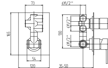
Mixer doccia da incasso 4 vie con deviatore Built-in 4-way shower mixer with diverter Смеситель скрытого монтажа 4х позиц.
