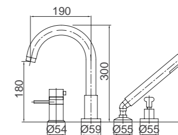
Batteria bordo vasca con doccia estraibile, termostato Bathtub set with pull-out shower, thermostatic Смеситель на борт ванны на 4 отверстия термостатический
