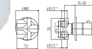
FORTIS 4 vie deviatore Built-in 4-way diverter Девiator 4х позиционный
