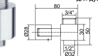
Prese acqua per la colonna doccia Fitting for shower column Штуцер проходной для душевой колонны
