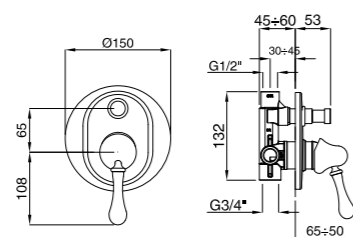
Mixer doccia da incasso 2 vie con deviatore Built-in 2 way shower mixer with diverter Смеситель скрытого монтажа с девиатором
