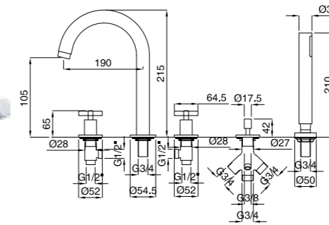
Batteria bordo vasca con doccia estraibile Bathtub set with pull-out hand shower Смеситель на борт ванны на 5 отверстий
