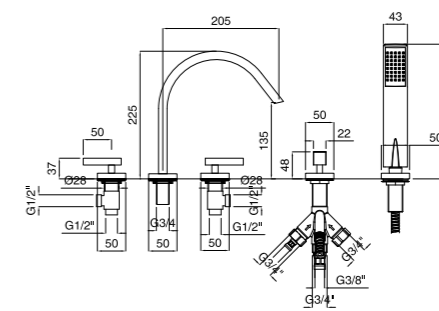
Batteria bordo vasca con doccia estraibile Bathtub set with pull-out hand shower Смеситель на борт ванны на 5 отверстий
