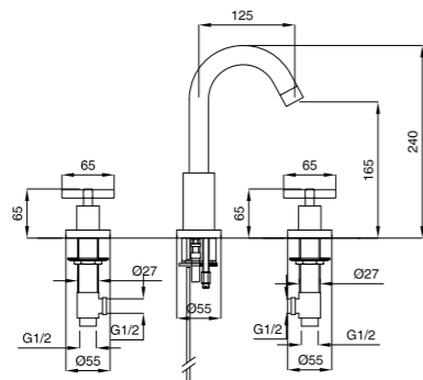
Batteria lavabo Washbasin mixer Смеситель для раковины на 3 отверстия
