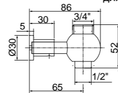
Prese acqua per la colonna doccia Fitting for shower column Штуцер проходной для душевой колонны
