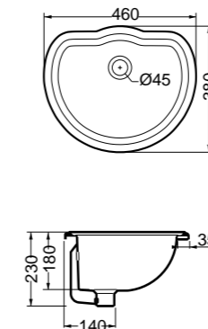
Lavabo Washbasin Раковина 46x38 см
