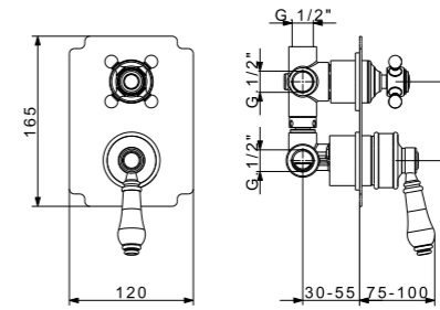
Mixer doccia da incasso 3 vie con deviatore Built-in 3 way shower mixer with diverter Смеситель скрытого монтажа с девиатором 3-х позиционный
