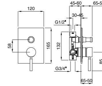
Mixer doccia da incasso 2 vie con deviatore Built-in 2 way shower mixer with diverter Смеситель скрытого монтажа, 2-х позиционный с девиатором
