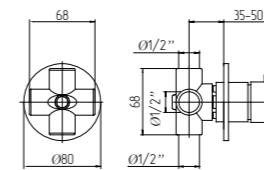
FORTIS 3 vie deviatore Built-in 3-way diverter Девiator 3х позиционный
