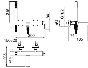
Monocomando vasca esterno con duplex External single lever bath mixer with duplex Смеситель для ванны монокомандный
