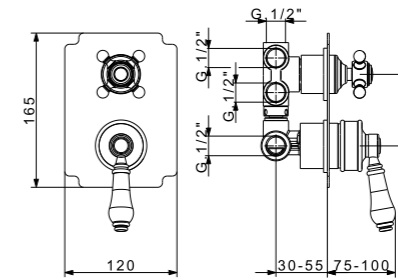
Mixer doccia da incasso 4 vie con deviatore Built-in 4 way shower mixer with diverter Смеситель скрытого монтажа с девиатором 4-х позиционный
