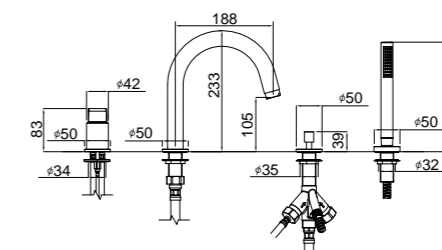
Batteria bordo vasca con doccia estraibile Bathtub set with pull-out shower Смеситель на борт ванны, монокомандный на 4 отверстия
