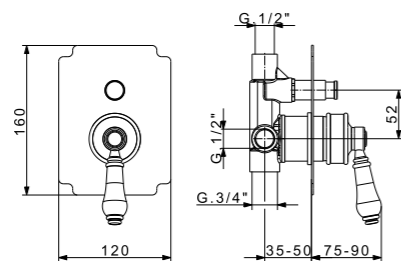
Mixer doccia da incasso 2 vie con deviatore Built-in 2 way shower mixer with diverter Смеситель скрытого монтажа с девиатором
