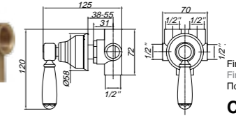
3 vie deviatore Built-in 3-way diverter Девiator 3х позиционный
