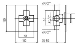
KVANT 3 vie deviatore Built-in 3-way diverter Девiator 3х позиционный
