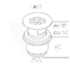
Scarico con troppopieno Pop-up waste with overflow Донный клапан под перелив
