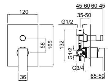
Mixer doccia da incasso 2 vie con deviatore Built-in 2 way shower mixer with diverter Смеситель моноком. скрытого монтажа, 2-х позиционный с девиатором
