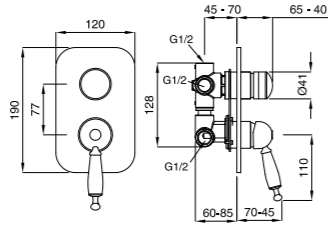
Mixer doccia da incasso 3 vie con deviatore Built-in 3 way shower mixer with diverter Смеситель 3-х позиционный с девиатором
