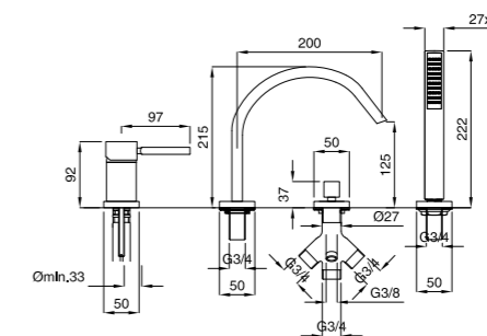
Batteria bordo vasca con doccia estraibile Bathtub set with pull-out hand shower Смеситель на борт ванны на 4 отверстия
