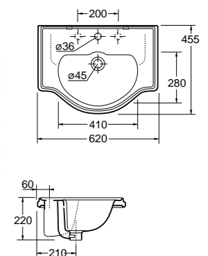
Lavabo Washbasin Раковина 62x46 см
