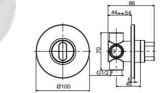
FORTIS 4 vie deviatore Built-in 4-way diverter Девiator 4х позиционный
