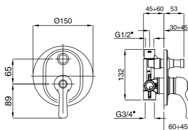
Mixer doccia da incasso 2 vie con deviatore Built-in 2 way shower mixer with diverter Смеситель скрытого монтажа с девиатором
