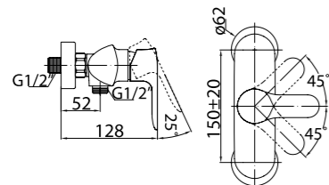
REN-ESDM-CRM Смеситель для душа
