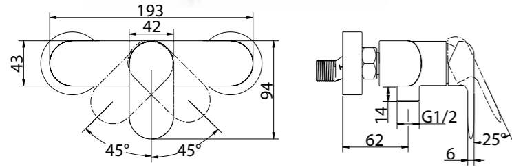
FER-ESDM-CRM Смеситель для душа
