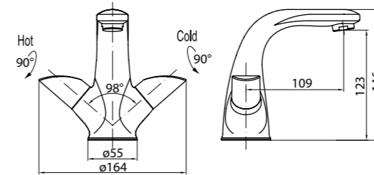
TIA-LV-CRM/TWIST Смеситель на раковину
