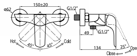
NOT-ESDM-CRM Смеситель для душа
