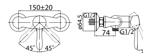
OGL-ESD-CRM Смеситель для душа
