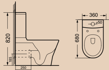
Унитаз компакт BB0118WP | BB0118BT | BB0118SC Чаша унитаза Бачок Сиденье
