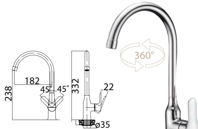
REN-LAM25-CRM Смеситель для кухни, D25
