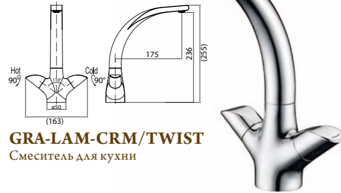
GRA-LV-CRM/TWIST Смеситель на раковину
