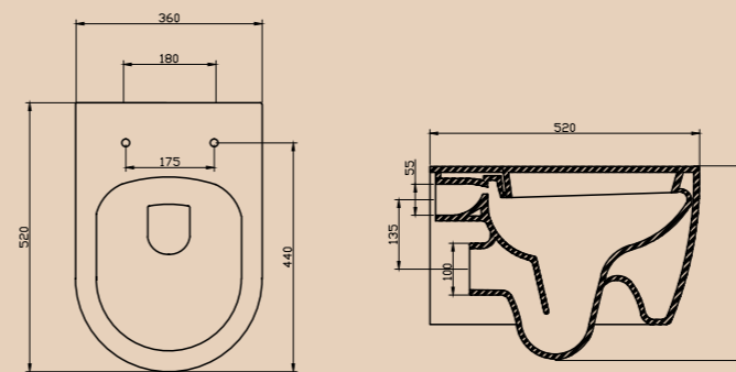
Унитаз подвесной BB105CH | BB105SC Чаша унитаза | Сидение
