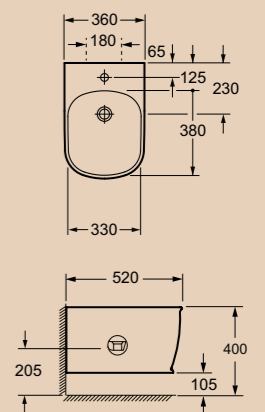
Биде подвесное BB10150BH Биде
