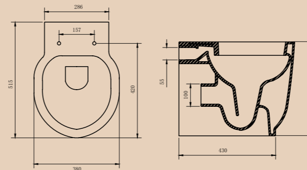
Унитаз приставной BB122CB | BB122SC Чаша унитаза | Сидение
