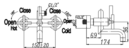
VIT-VAS-CRM Смеситель для ванны и душа
