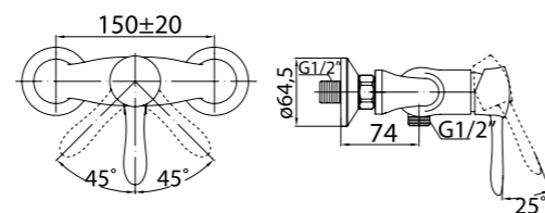
VOL-ESDM-CRM Смеситель для душа
