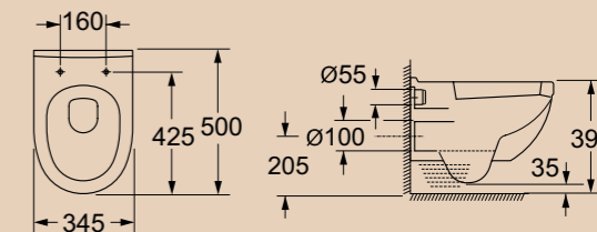
Унитаз подвесной BB1076CH | B1076SC Чаша унитаза | Сиденье
