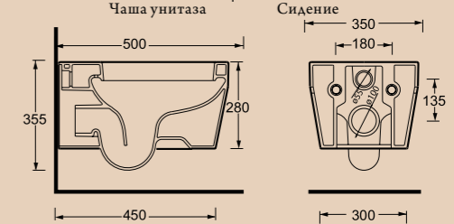
Унитаз подвесной BB540CH | BB540SC Чаша унитаза | Сидение
