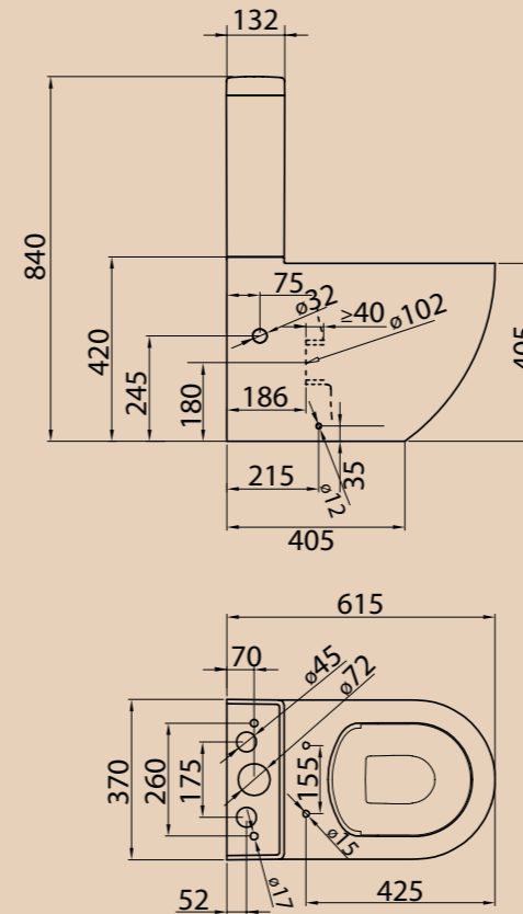
Унитаз компакт безободковый BB006CPR | BB006T | BB2019SC Чаша унитаза | Бачок | Сидение
