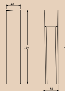
Раковина на пьедестале BB540L | BB540P Чаша раковины | Пьедестал
