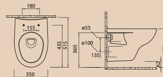
Унитаз подвесной BB9363CH | BB9363SC Чаша унитаза | Сиденье
