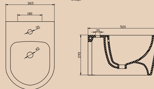
Биде подвесное BB105BH Биде
