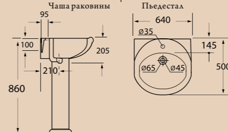
BB1078L | BB1078P Чаша раковины | Пьедестал
