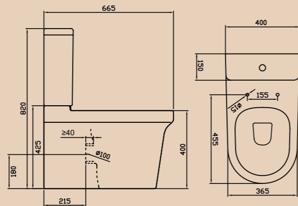
Унитаз компактный BB829CP | BB829T | BB2019SC Чаша унитаза | Бачок | Сиденье
