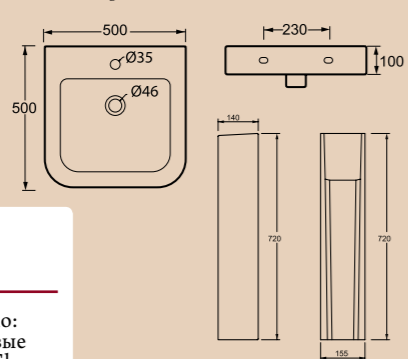
BB540L | BB540P Чаша раковины | Пьедестал
