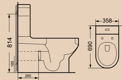
Унитаз компакт BB0121WP | BB0121T | BB0121SC Чаша унитаза | Бачок | Сидение
