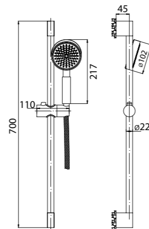
VIT-SAL-CRM Душевой гарнитур
