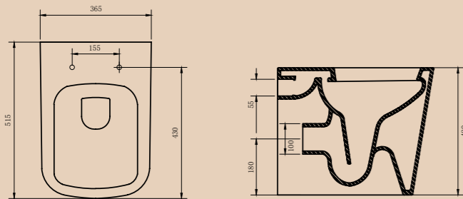
Унитаз приставной BB120CB | BB120SC Чаша унитаза | Сидение
