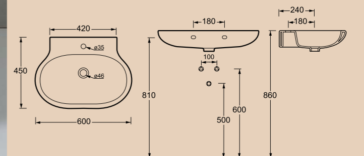
Раковина на пьедестале BB548BL | BB548P Чаша раковины | Пьедестал
