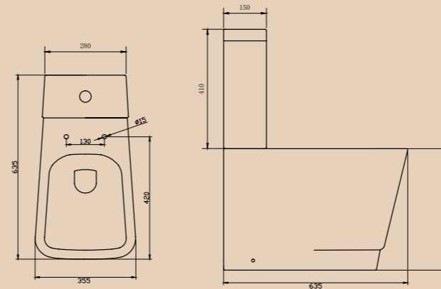
Унитаз компакт BB121CP | BB121T | BB121SC Чаша унитаза | Бачок | Сидение
