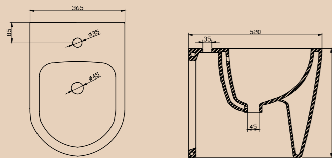
Биде напольное BB105B Биде
