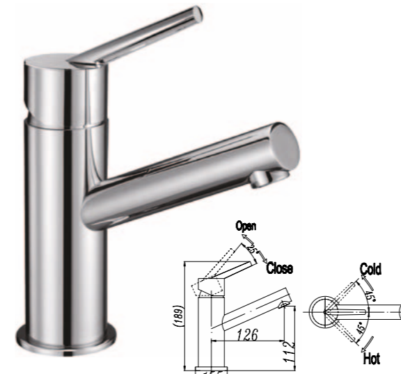
ISO-LVM-CRM Смеситель на раковину
