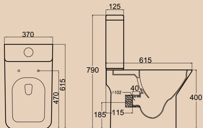
Унитаз компакт BB353CPR | BB353T | BB353SC Чаша унитаза | Бачок | Сидение
