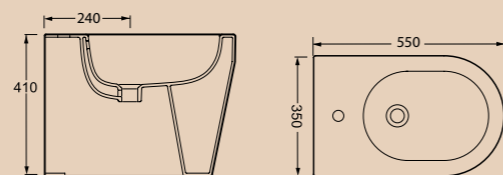
Биде BB541B Биде
