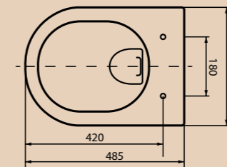
Унитаз подвесной VITALE BB037CH | BB2009SC Чаша унитаза | Сидение
