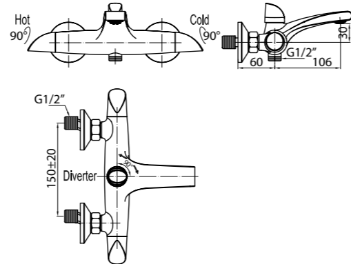
GRA-VAS-CRM/TWIST Смеситель для ванны и душа (ручной душ со шлангом приобретается отдельно)
