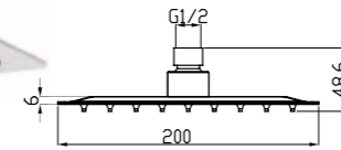
BB-SLD2C-200-CRM Верхний душ, 20x20 см
