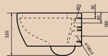
Унитаз подвесной VITALE BB037CH | BB2009SC Чаша унитаза | Сидение
