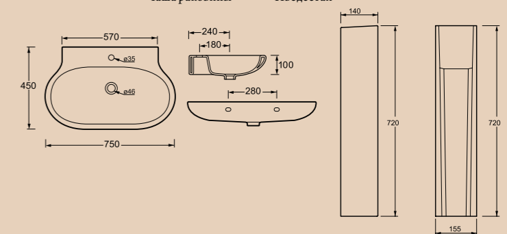
Раковина на пьедестале BB548BL | BB548P Чаша раковины | Пьедестал
